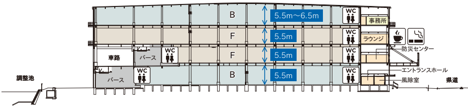
A-A'断面図
