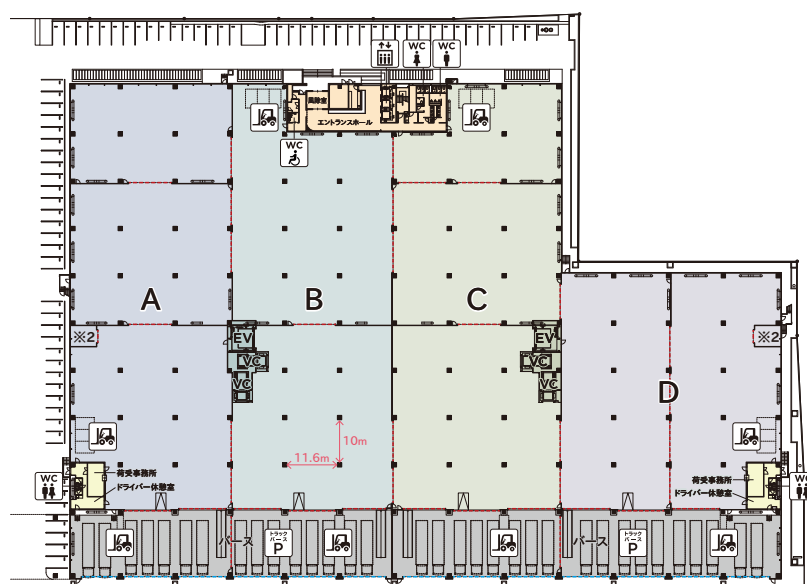
1F平面図
