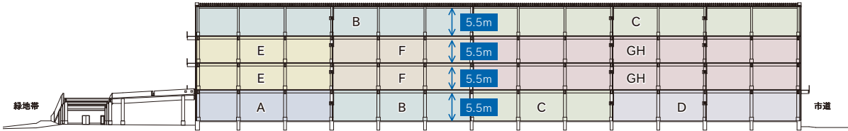
B-B'断面図
