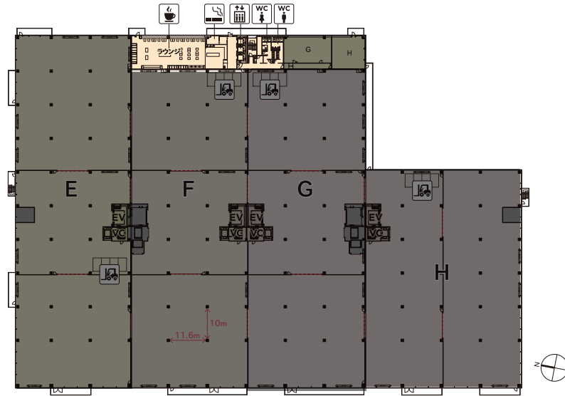
3F平面図
