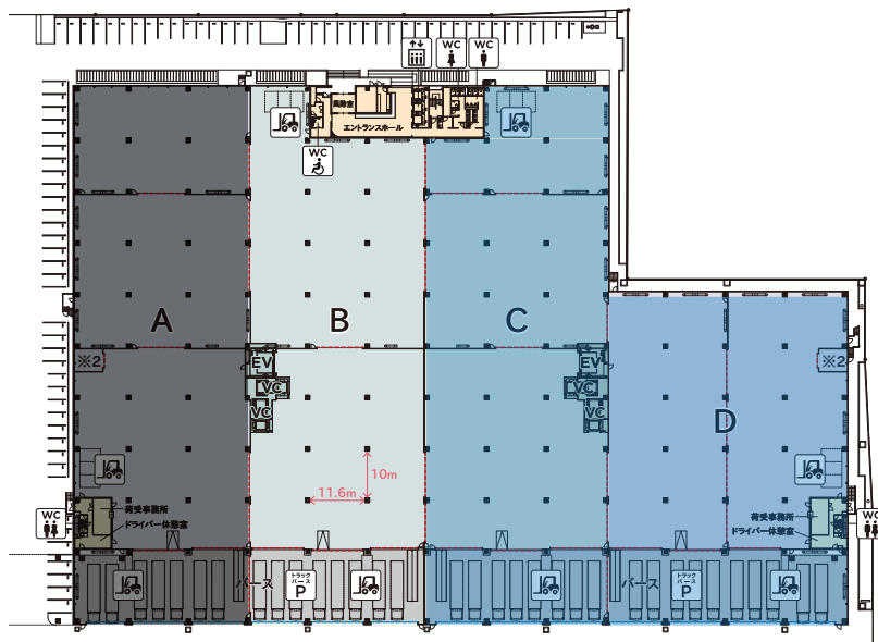
1F平面図
